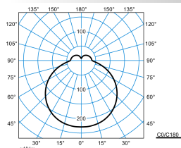
Mondia G3 Z WD3 DW 32-840 ET2
