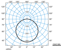
Olisq RWD3 DW 30-840 ETBLE +DMM IP54 + Olisq RWD3 C 01
