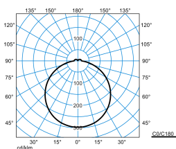
Olisq RWD3 DW 30-840 ETBLE +DMM IP54 + Olisq RWD3 ZDR 1/2 01
