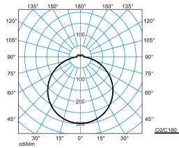
Olisq RWD3 DW 30-840 ETBLE +DMM IP54
