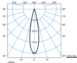
7651 LentyP L-SP 30-827 M32 ET 01 (150)
