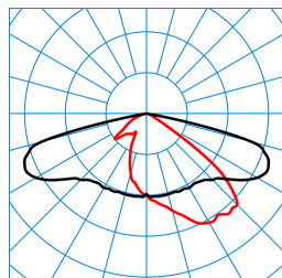
LIQ 70N-AB7L-LR/6800-722 8G1 ET (CLO end value) TX778273 ■ C0 - C180 ■ C90 - C270 DIN 5040: A30 UTE: 1,00 E DLOR: 100 % ULOR: 0 % CEN Flux Code: 39 76 98 100 100
