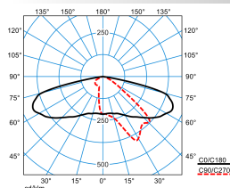
Jovie 50-AB2L-ML-LR/1000-2200-730 2G1 ET (CLO initial value)
