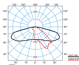
Jovie 50-AB2L-ML-LR/1000-2200-730 2G1 ET (CLO end value)
