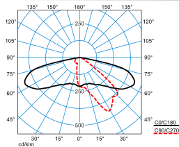
Publisca P3-AB2L-LR/2200-730 2G1
