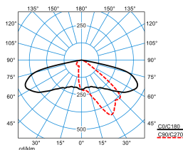
Publisca P3-AB2L-LR/2200-730 2G1 ET (CLO initial value)
