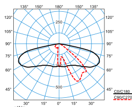
Publisca P2-AB2L-LR/1100-730 2G1S ET (CLO end value)
