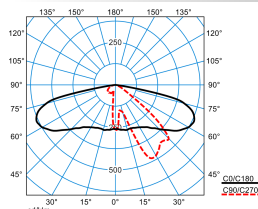
Publisca P2-AB2L-LR/1100-730 2G1S ET (CLO initial value)
