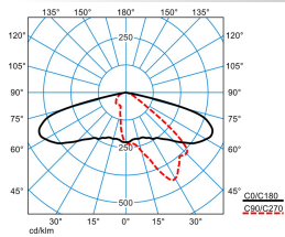
Jovie 50-AB2L-6-68-730-CLO-B
