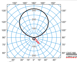
Luceos S G3 PAW-IL 170-9TW ETDS FT 03 (DWW)
