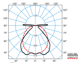
AragF 15 PW 27-88/16ML-840 ET (stage 5)
