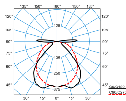
AragF 15 PW 27-88/16ML-840 ET (stage 4)
