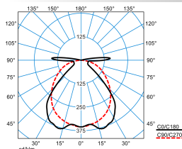
AragF 15 PW 27-88/16ML-840 ET (stage 0)
