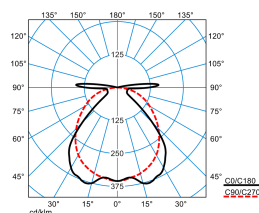
AragF 15 PW 27-88/16ML-840 ET (stage 3)
