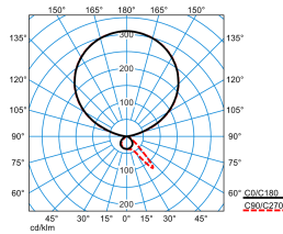
Luceos S BS G3 PAW-IL 125-830 ETDS FT 01
