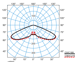
Publisca P2-RB6L-LR/4200-730 6G1S ET (CLO end value)
