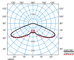
Publisca P2-RB6L-LR/4200-730 6G1S ET (CLO initial value)
