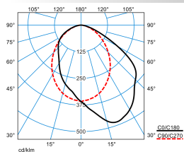
Opendo D1-L DWW 42-840 ET 03 TX277444
