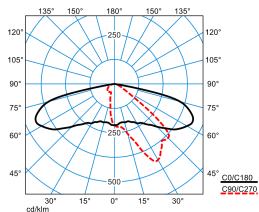
Publisca P3-AB2L-LRA/1800-740 4G1 ET (CLO end value)
