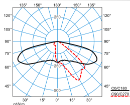
Publisca P3-AB2L-LRA/1800-740 4G1 ET (CLO initial value)
