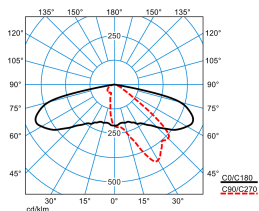
Publisca P3-AB2L-LRA/1800-740 4G1
