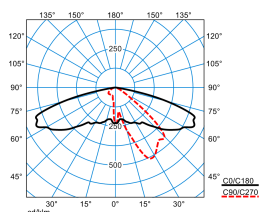
Publisca P1W-AB2L-LRA/4600-730 6G1S
