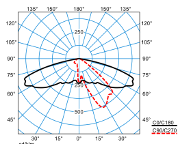
Publisca P1W-AB2L-LRA/4600-730 6G1S ET (CLO end value)
