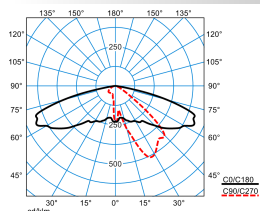
Publisca P1W-AB2L-LRA/4600-730 6G1S ET (CLO initial value)
