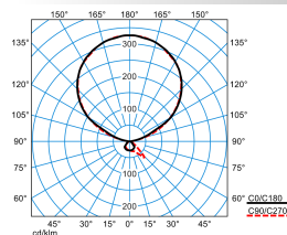
Luceos S G2 PAW-IL 85-830 ETDD 01
