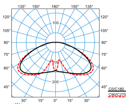
Publisca P1W-RBT-LR/1800-740 2G1S ET (CLO end value)
