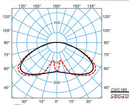
Publisca P1W-RBT-LR/1800-740 2G1S ET (CLO initial value)
