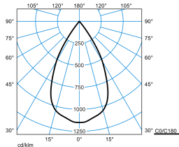
E-Line PRO 78 BV G2 RF-VFL 50-830 M33 ETDD 03 03
