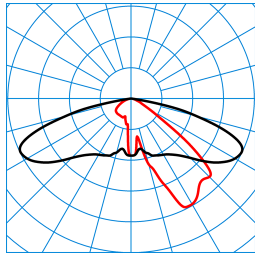
Publisca P2-AB2L/5600-740 6G1S ETDD (CLO end value) TX300307 ■ C0 - C180 ■ C90 - C270 DIN 5040: A30 UTE: 1,00 G DLOR: 100 % ULOR: 0 % CEN Flux Code: 35 74 97 100 100
