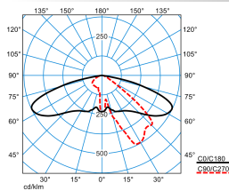
Publisca P2-AB2L/5600-740 6G1S
