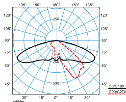
Publisca P2-AB2L/5600-740 6G1S ETDD (CLO end value)
