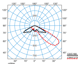
LnPlus 40-AM19L-SLR1/5100-740 6G1 ET (CLO end value)
