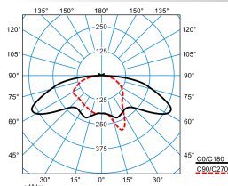
9811IA-LRA/2200-840 ET
