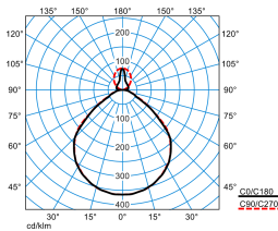
Luceos D/H1-L CDP 4000-8TW ETDD 03 (Ceiling D1 ZD/03) (DCW)
