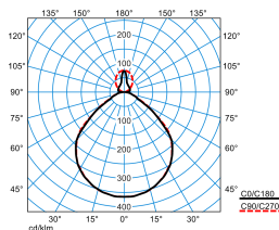
Luceos D/H1-L CDP 4000-8TW ETDD 03 (Ceiling D1 ZD/03) (DSU)
