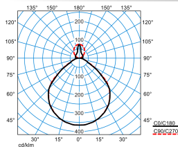
Luceos D/H1-L CDP 4000-8TW ETDD 03 (Ceiling D1 ZD/03) (DWW)
