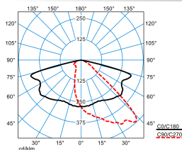
Cuvia 60-AB6L-LRA/5600-740 8G1S ET
