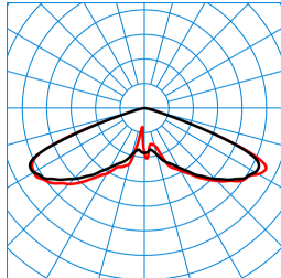
Publisca P2-RB6L-LR/2400-740 3G1S TX047861 ■ C0 - C180 ■ C90 - C270 DIN 5040: A20 UTE: 1,00 J DLOR: 100 % ULOR: 0 % CEN Flux Code: 20 57 98 100 100
