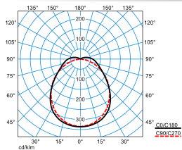
OleveonF 12 L 4000-840 ET +HFS TX770697
