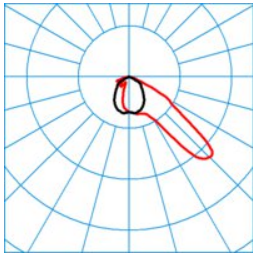
Jovie 50-AM2L-4-32-740-CLO-E
