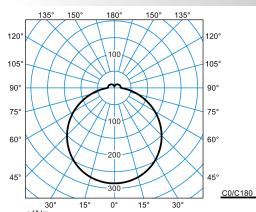
Olisq RWD2 DW 40-8TW ETBLE +CAS IP54 (DWW)
