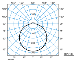
Olisq RWD2 DW 40-8TW ETBLE +CAS IP54 (DCW)
