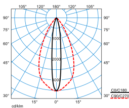
Altigo G2 90 SE6L/3000-830 1G1P + VE IP66 24V DC 60W
