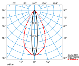
Altigo G2 90 SE6L/3000-830 1G1P + VE IP66 24V DC 130W
