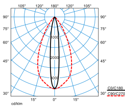
Altigo G2 90 SE6L/3000-830 1G1P + G2 VE IP66 24V DC 80W
