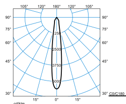
E-Line PRO 78 BV G2 RF-SP 40-840 M35 ET 05 05
