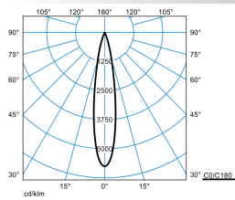
LentyEB L-SP 20-EW M61 ET 05
