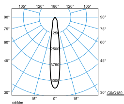
E-Line PRO 78 BV G2 RF-SP 20-827 M32 ET 01 Blank
