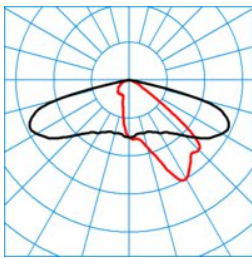
Jovie 50-AB2L-4-42-740-CLO-B
