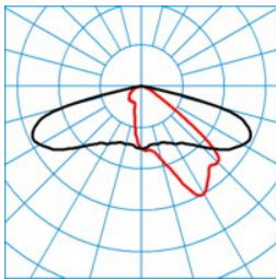
Jovie 50-AB2L-4-42-740-CLO-E
