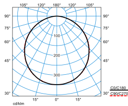
Olisq QWD3 DW 30-830 ET IP54 + Olisq QWD3 ZDR 1/1 05
