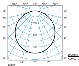
Olisq QWD3 DW 30-830 ET IP54 + Olisq QWD3 ZDR 1/1 01
