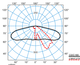
Publisca P1-AB2L-LRA/1100-730 2G1S ET (CLO end value) TX301300 DIN 5040: A30 UTE: 1,00 G DLOR: 100 % ULOR: 0 % CEN Flux Code: 34 70 96 100 100
