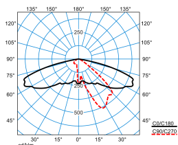
Publisca P1W-AB2L-LR/3800-730 6G1S ET (CLO end value)
