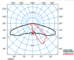
Publisca P1W-AB2L-LR/3800-730 6G1S
