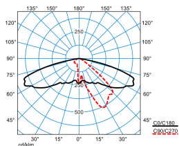
Publisca P1W-AB2L-LR/3800-730 6G1S ET (CLO initial value)
