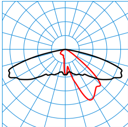
Publisca P1W-AB2L-LR/3800-730 6G1S TX053487 ■ C0 - C180 ■ C90 - C270 DIN 5040: A30 UTE: 1,00 G DLOR: 100 % ULOR: 0 % CEN Flux Code: 34 72 97 100 100 0 0 0 0
