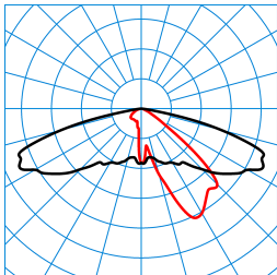
Publisca P1W-AB2L-LR/3800-730 6G1S ET (CLO end value) TX301438 ■ C0 - C180 ■ C90 - C270 DIN 5040: A30 UTE: 1,00 G DLOR: 100 % ULOR: 0 % CEN Flux Code: 34 72 97 100 100 0 0 0 0
