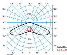
Publisca P2-RB6L-LR/1000-740 2G1S ET (CLO end value)
