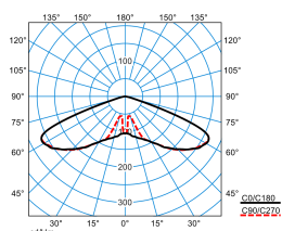
Publisca P2-RB6L-LR/1000-740 2G1S ET (CLO initial value)
