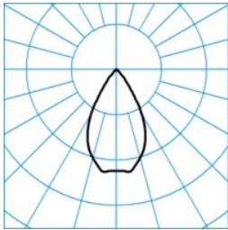
SNS QC7-MR1VFL-26-830
