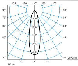
SisC 1Z RF-MF 50-840 M35 ETDD 05
