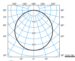
Olisq RWD4 DW 60-840 ETDD + Olisq RWD4 ZDR 1/1 05
