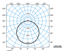
Olisq RWD4 DW 60-840 ETDD + Olisq RWD4 ZDR 1/2 03
