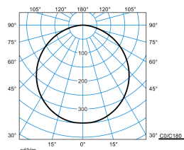
Olisq RWD4 DW 60-840 ETDD + Olisq RWD4 ZDR 1/1 01
