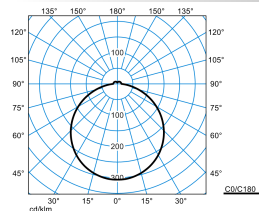
Olisq RWD4 DW 60-840 ETDD
