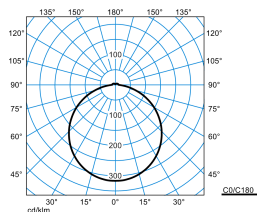
Olisq RWD4 DW 60-840 ETDD + Olisq RWD4 ZDR 1/2 05
