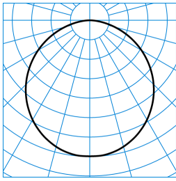
Olisq RWD4 DW 60-840 ETDD + Olisq RWD4 ZDR 1/1 01 TX427223
