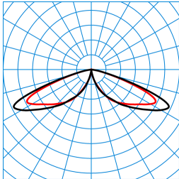
LTX ZT-RB6L-LRA/1200-740 2G1 ETDD TX779384
