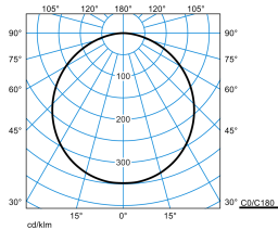
Olisq RWD2 DW 20-840 ETDD IP54 PC + Olisq RWD2 ZDR 1/1 03
