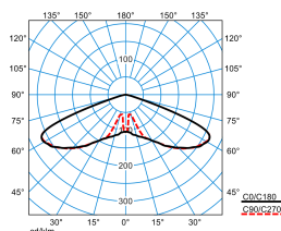
Publisca P1-RB6L/1200-730 2G1S
