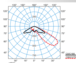
LnPlus 40-AM19L-SLR1/15000-730 12G1 ET (CLO initial value)
