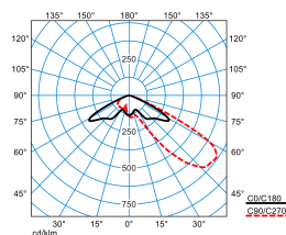
LnPlus 40-AM19L-SLR1/15000-730 12G1 ET (CLO end value)
