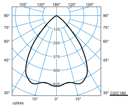
InperiaLP C05 BR22 1000-840 ET 03
