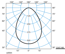
InperiaLP C05 BR22 1000-840 03 + DA-M 03
