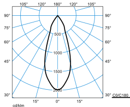
E-Line PRO 78 BV G2 RF-FL 40-EW M48 ETDD 03 Blank
