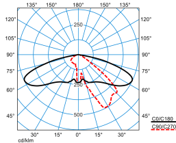
Publisca P1-AB2L-LR/5600-740 6G1S TX047539 DIN 5040: A30 UTE: 1,00 G DLOR: 100 % ULOR: 0 % CEN Flux Code: 35 74 97 100 100
