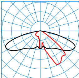
Publisca P1-AB2L-LR/5600-740 6G1S ET (CLO end value) TX301111 ■ C0 - C180 ■ C90 - C270 DIN 5040: A30 UTE: 1,00 G DLOR: 100 % ULOR: 0 % CEN Flux Code: 35 74 97 100 100
