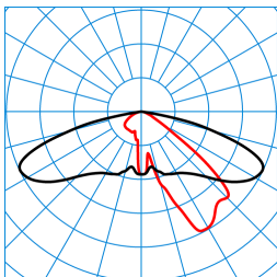
Publisca P1-AB2L-LR/5600-740 6G1S ET (CLO initial value) TX301752 ■ C0 - C180 ■ C90 - C270 DIN 5040: A30 UTE: 1,00 G DLOR: 100 % ULOR: 0 % CEN Flux Code: 35 74 97 100 100
