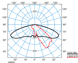
Publisca P1-AB2L-LR/5600-740 6G1S ET (CLO initial value)
