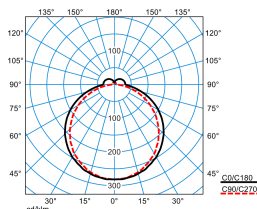
Olisq LWD1 DW 20-40/4/ML-830 ET IP54 IK (stage 2)
