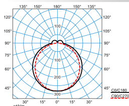
Olisq LWD1 DW 20-40/4/ML-830 ET IP54 IK (stage 1)
