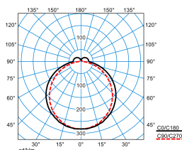
Olisq LWD1 DW 20-40/4/ML-830 ET IP54 IK (stage 4)
