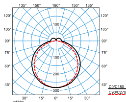
Olisq LWD1 DW 20-40/4/ML-830 ET IP54 IK (stage 3)
