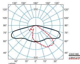
LIQ 70N-AB7L-LRA/7500-727 8G1 ETDD(CLO initial value)
