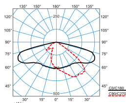
LIQ 70N-AB7L-LRA/7500-727 8G1 ETDD(CLO end value)
