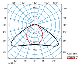
Nextrema G3 XB 6000-840 ETDD +HFSX LV PC
