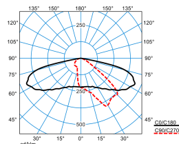
LIQ 50N-AB2L-LR/2000-722 2G1 ET (CLO end value)
